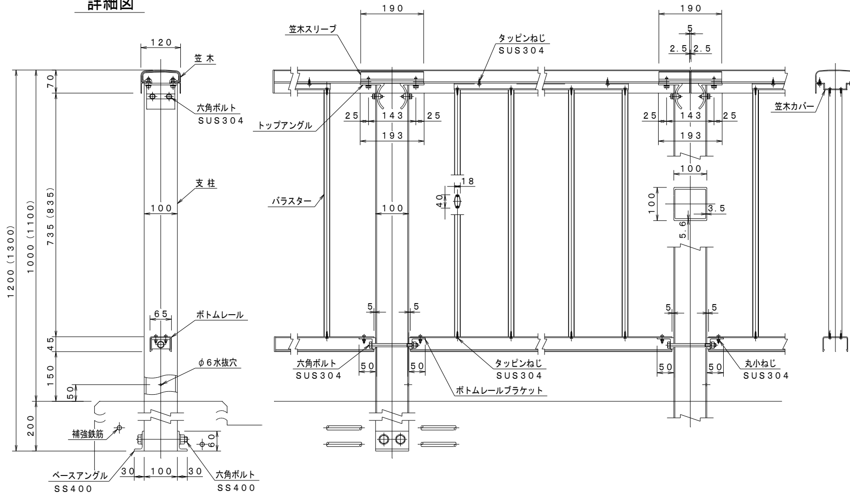
詳細図
